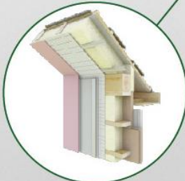
ZATEPLENIE POMŮRNICE
