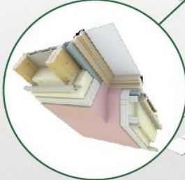
ZATEPLENIE STREŠNÉHO OKNA
