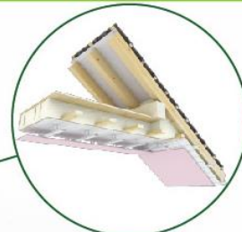
ZATEPLENIE ŠIKMEJ STRECHY NA DIFÚZNU FÓLIU
